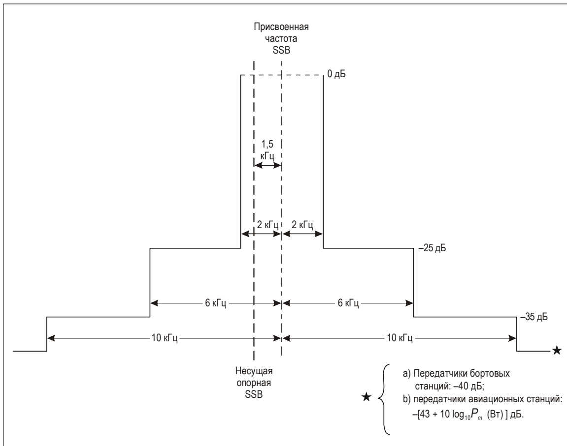
Рис. 2-1. Пределы спектра частот (выраженные через среднюю мощность), требуемые для всех типов передатчиков бортовых станций и передатчиков авиационных станций, впервые установленных до 1 февраля 1983 года
