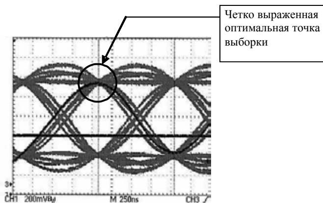
Рис. 12-3. Идеальная глазковая диаграмма
