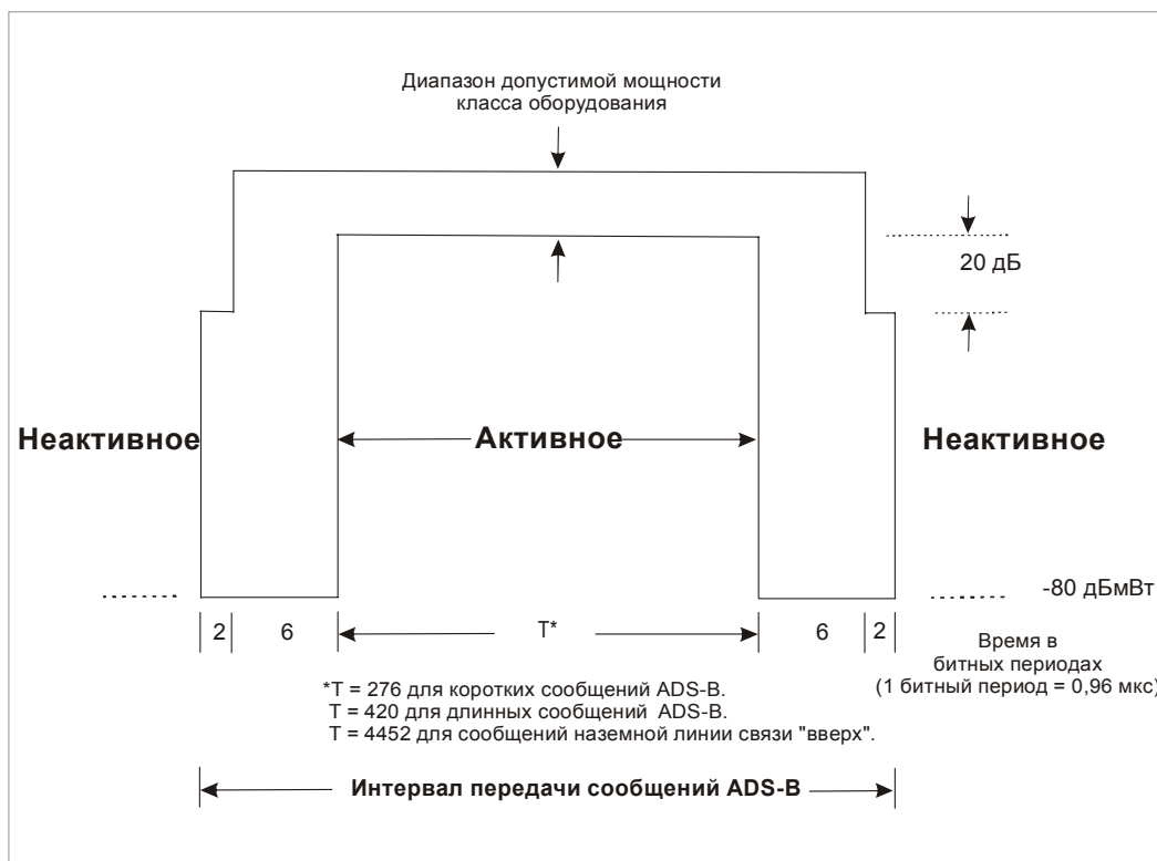
Рис. 12-2. Параметры времени/амплитуды передачи сообщений UAT
