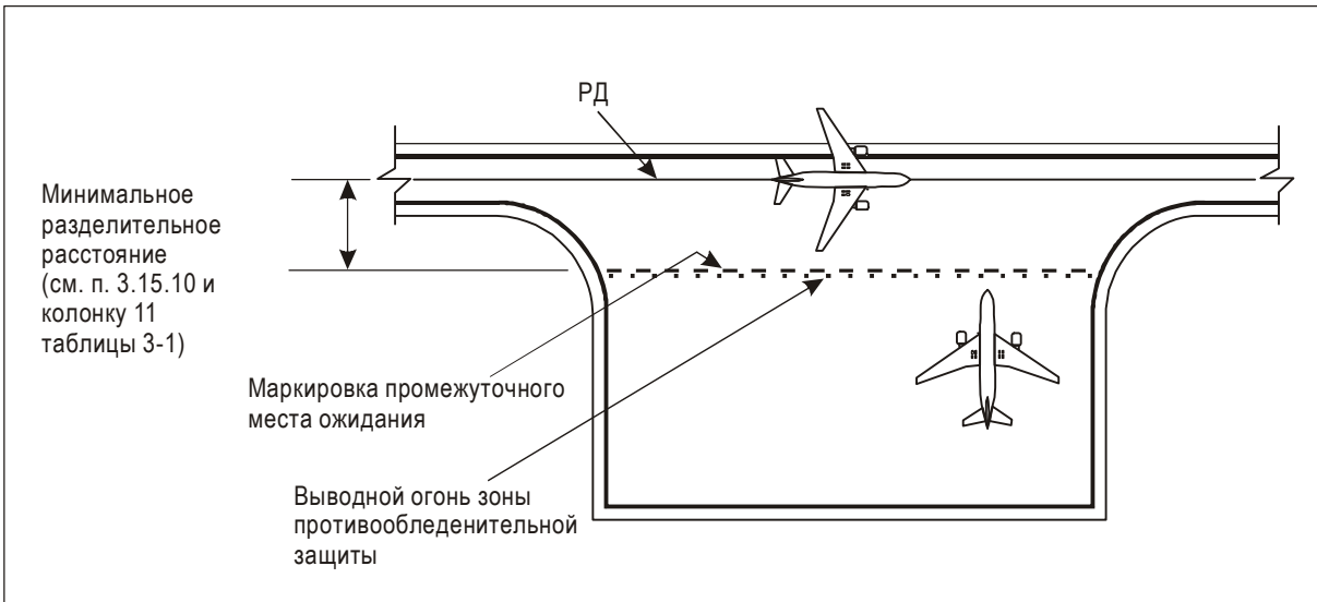
Рис. 5-28. Типичная удаленная зона противообледенительной защиты
