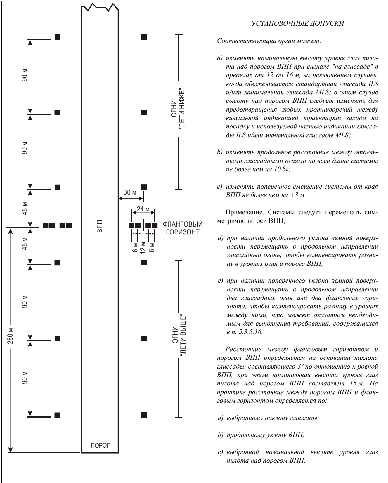
Рис. 5-17. Местоположение глиссадных огней системы T-VASIS
