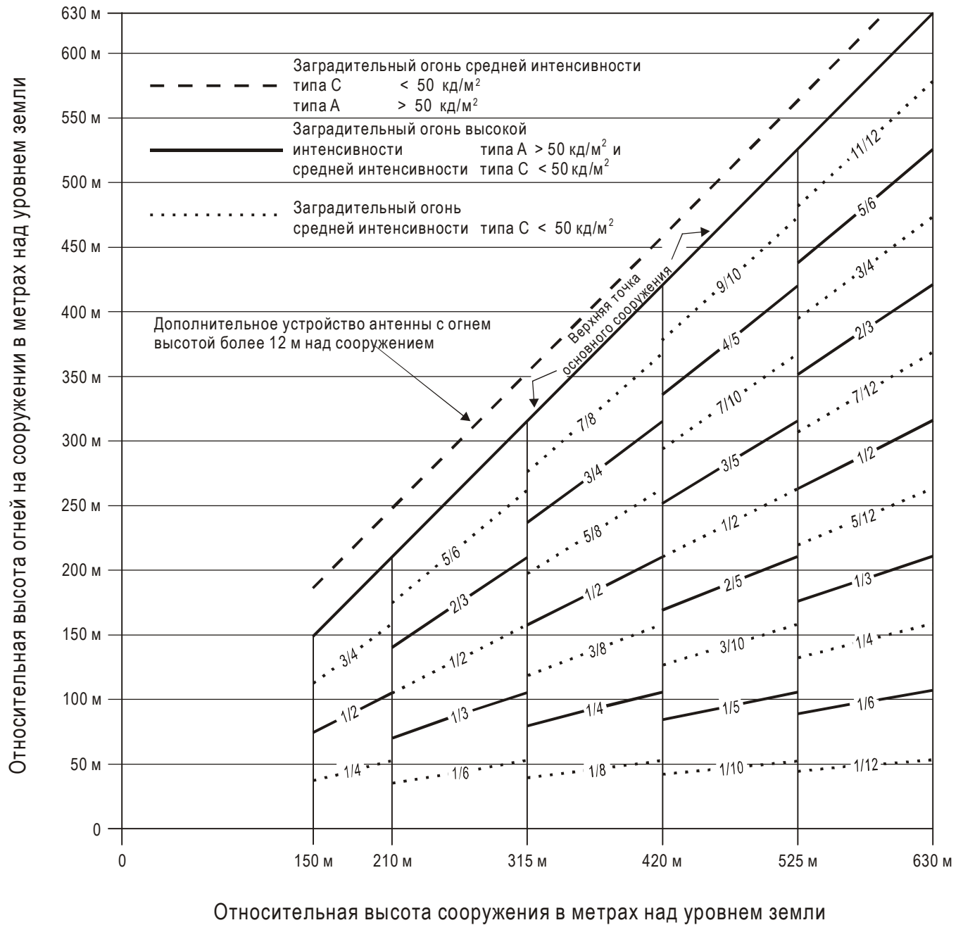
Рис. А6-8. Двойная система светоограждения препятствий с огнями высокой/средней интенсивности типа А/типа С
