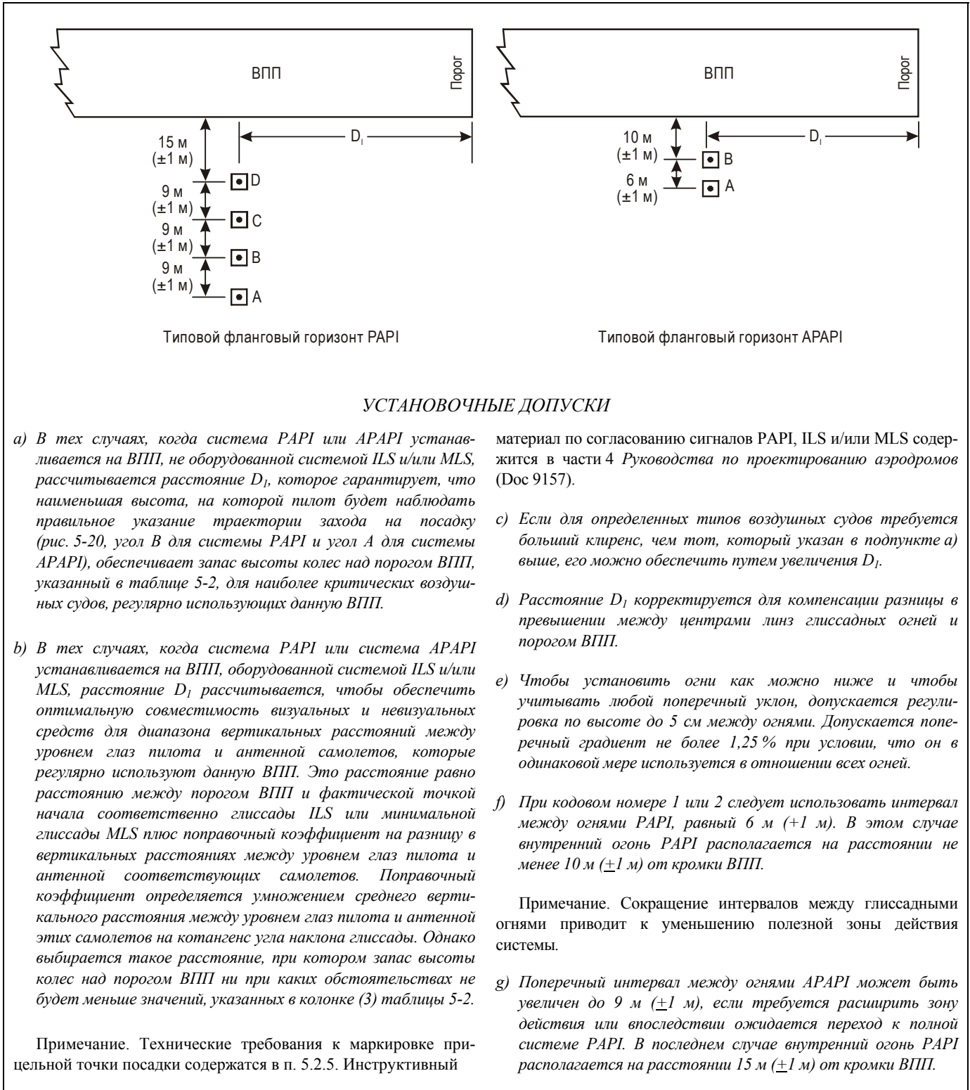
Рис. 5-19. Расположение PAPI и APAPI
